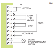
SPW11 (SMA1A)
